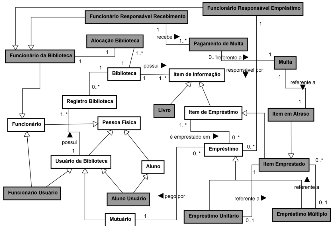
Figura 3.14 –Modelo de Integração (conceitos adicionais em destaque)
