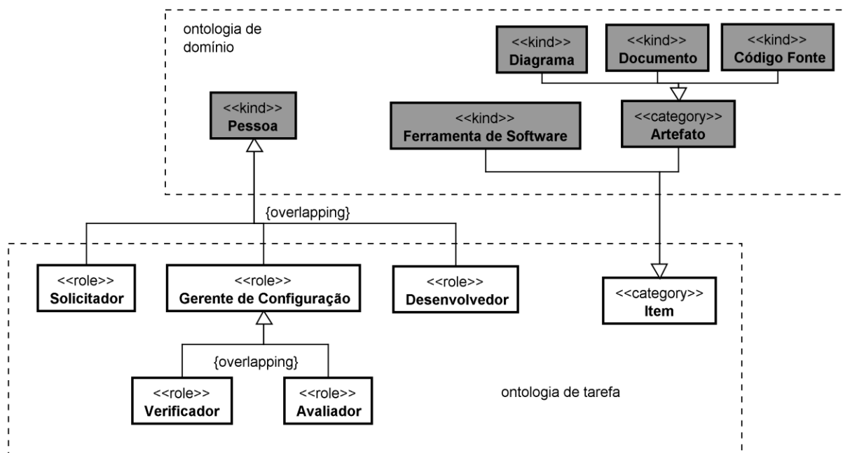
Figura 4.10– Ligação de complementação entre papéis da tarefa de GC e conceitos da GCS (representação dos papeis de conhecimento)
