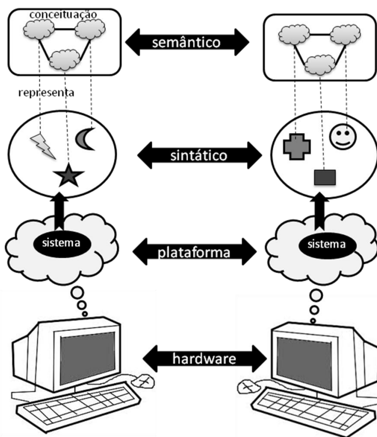
Figura 2.5 -Ilustração dos níveis de integração entre sistemas
